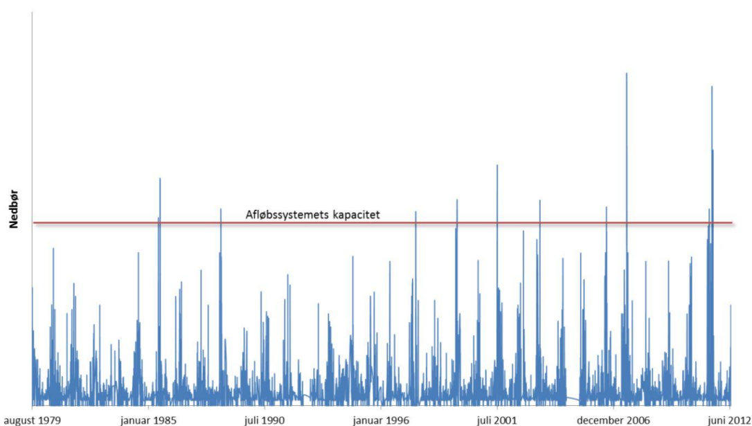
Figur 1.2. Regnvandsventiler kan skære toppen af de større regnskyl, inden de når kloakken
